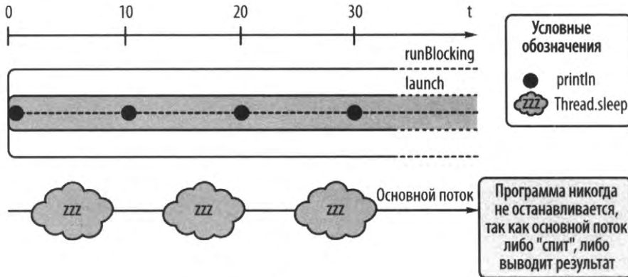
Рис. 7.2. Бесконечная программа
