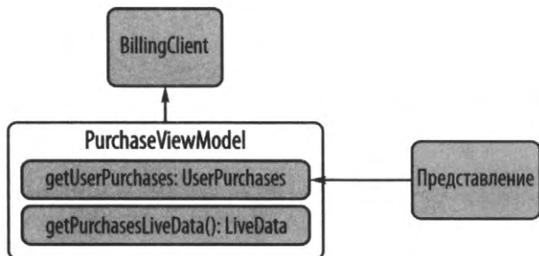
Рис. 6.1. Архитектура Model-View-ViewModel
