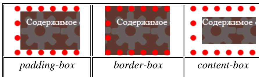
9.1-rasm. Turli qiymatlarni qo'llash natijasi
