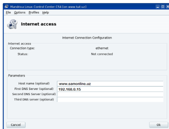
26.7-rasm. Ulanishlarni boshqarish.
