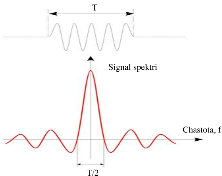
2.9- rasm. T davomiyligidagi simvol va uning spektri
