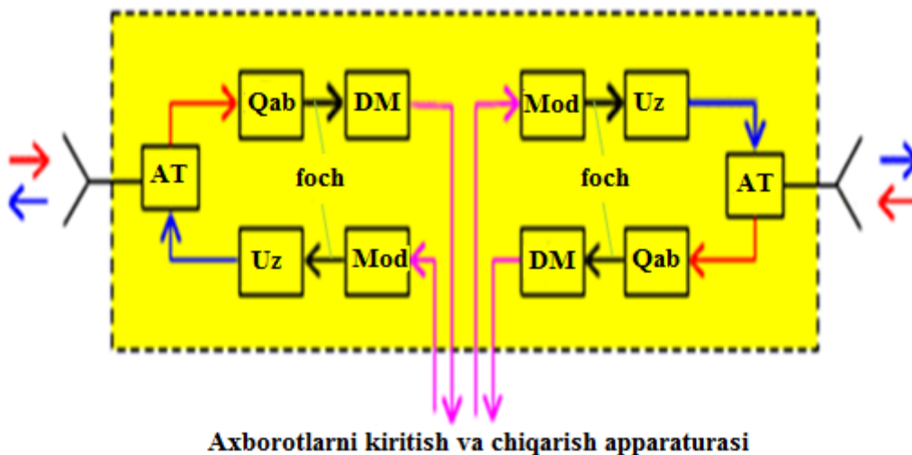
3.4- rasm. Uzel stansiyani tuzilish sxemasi
