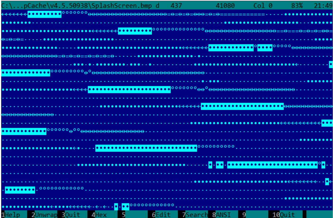
Рис. 5.15: Фрагмент BMP-файла
