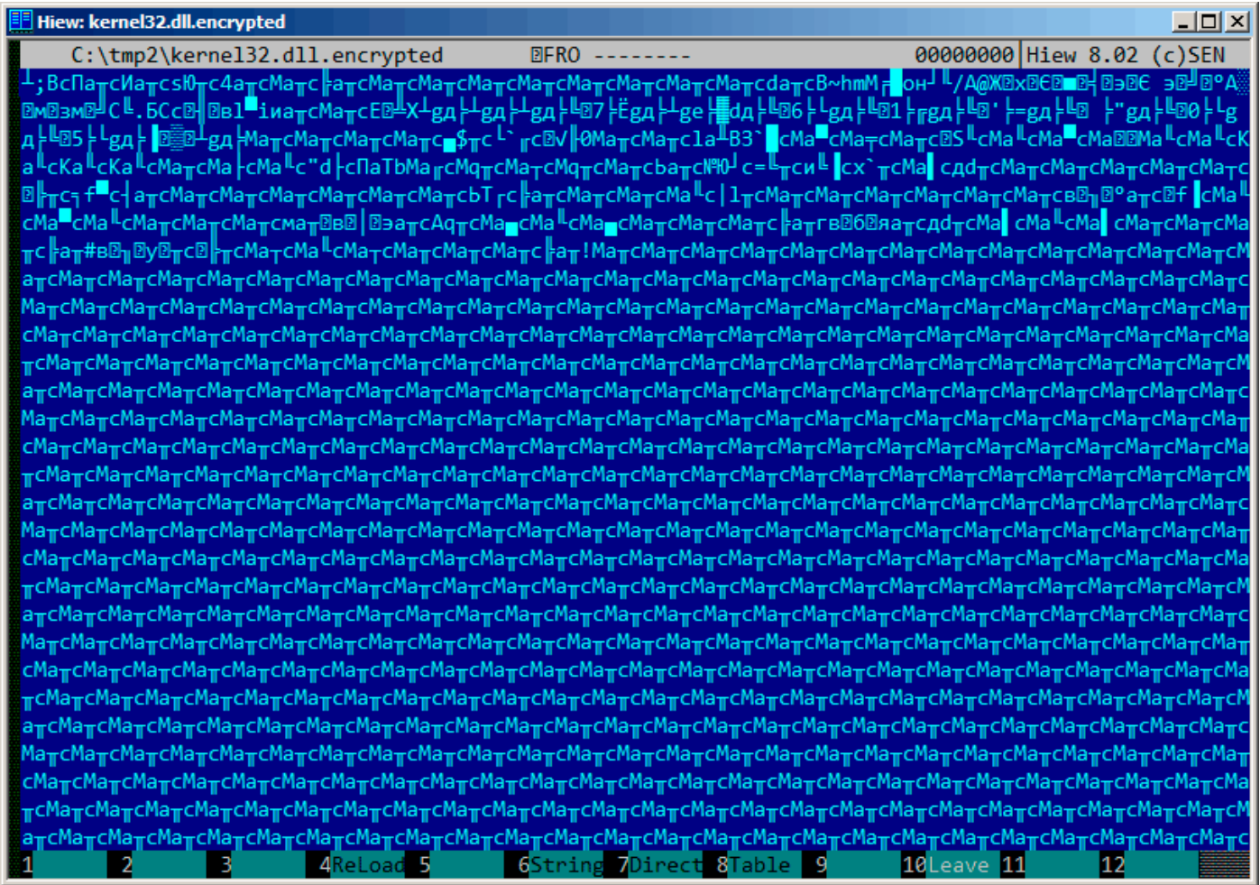
Рис. 9.4: «Зашифрованный» файл
