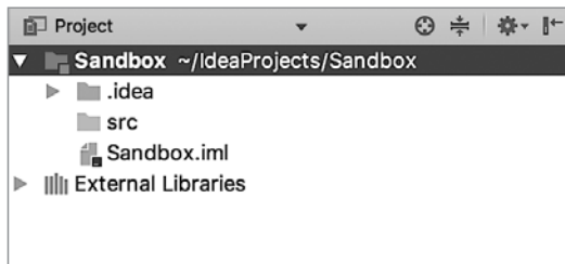
Рис. 1.7. Просмотр проекта
