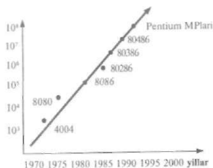
4.4.-rasm. Kompyuter mikroprotssessorlarining rivojlanib borishi bilan mikrochizmadagi tranzistorlarning ko'payishi tendensiyasi
