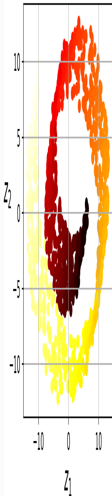
Linear kernel
