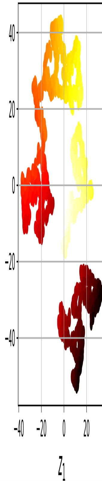
t-SNE
