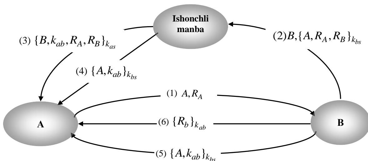
3.13- rasm. Yahalom protokoli
