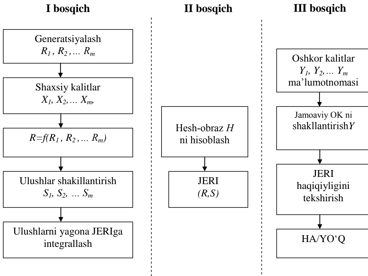
4.5- rasm. GOST R. 34.10-2001 va Shnorrr shemalari asosida JERI shakllantirish va tekshirish usuli
