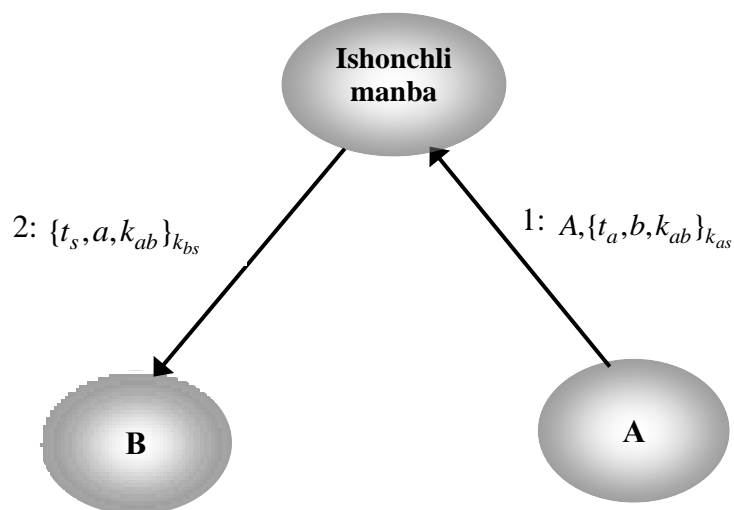
3.17- rasm. Katta halqumli qurbaqa protokoli
