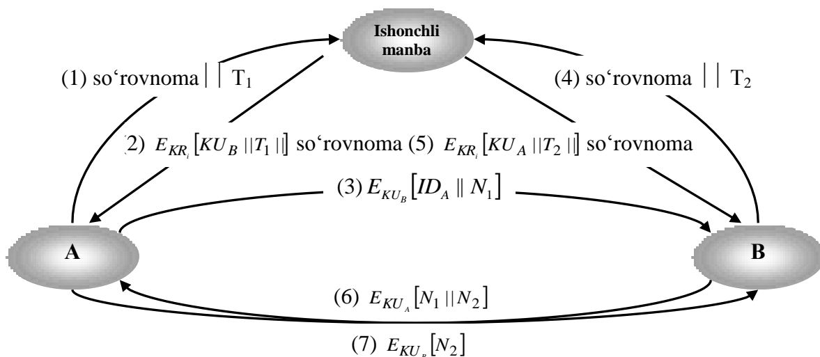
3.3- rasm. Ochiq kalitlarning ishonchli manbai
