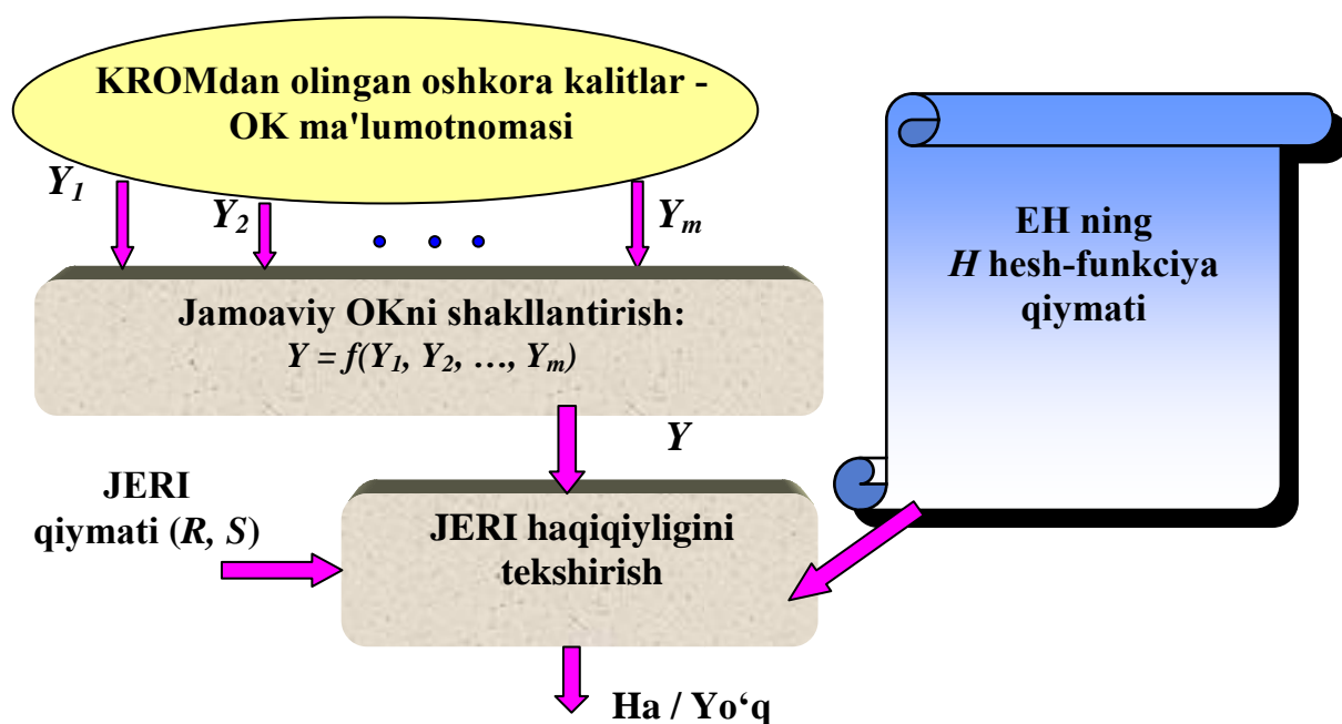
4.4- rasm. JERI haqiqiylikini tekshirishning umumiy shemasi
