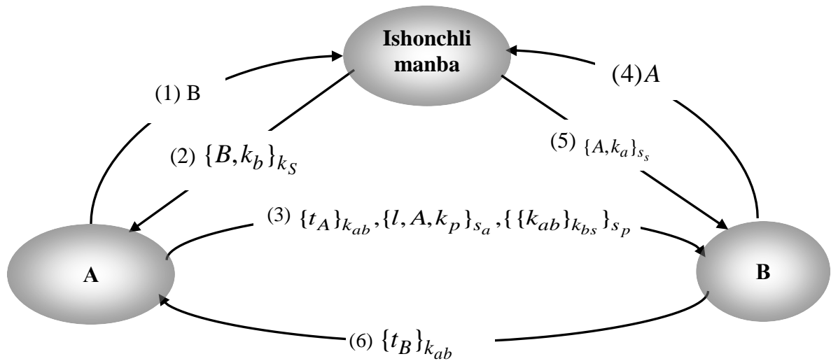
3.19- rasm. DASS protokoli
