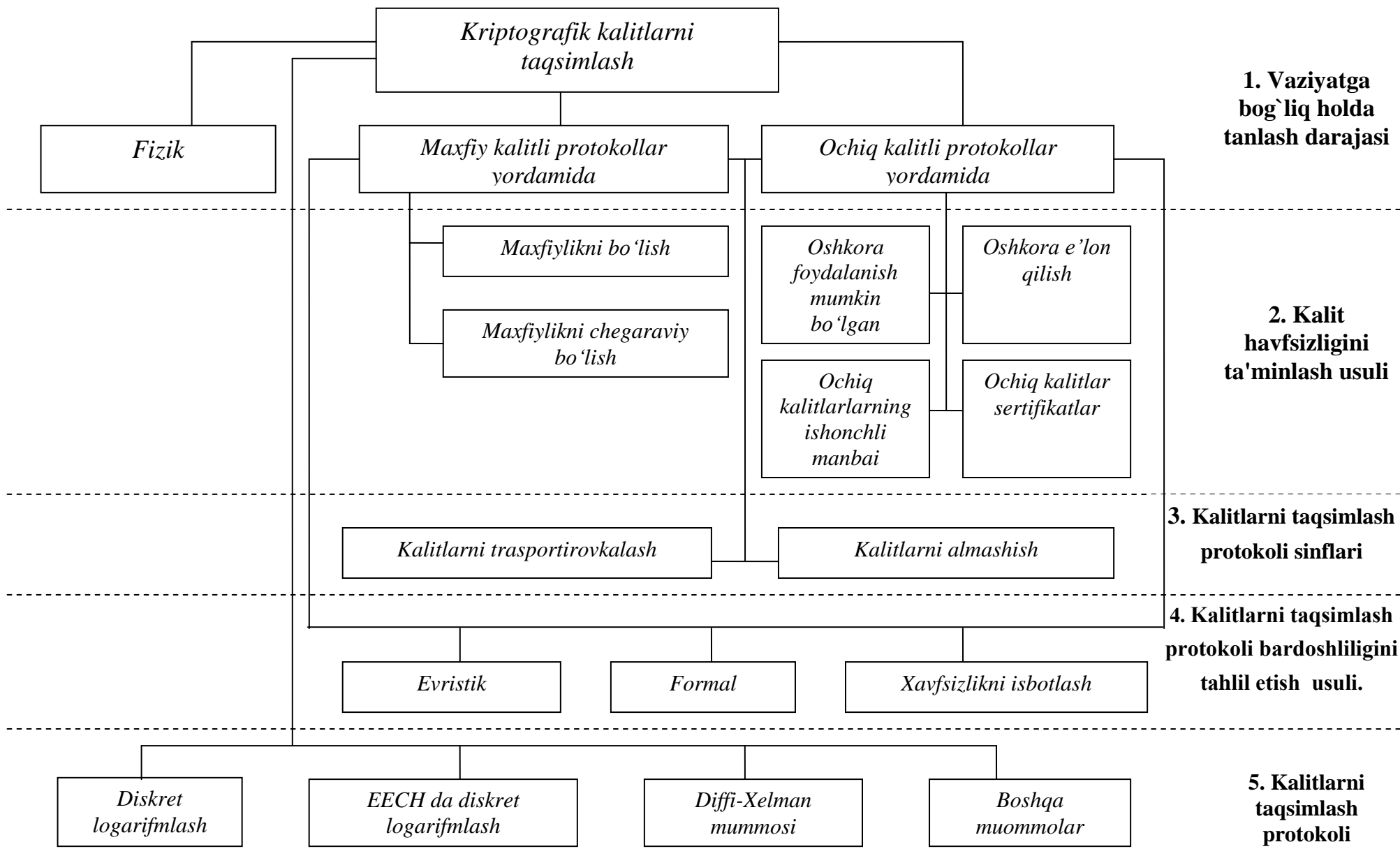
3.24- rasm. Kriptografik kalitlarni taqsimlash usullari tasnifi
