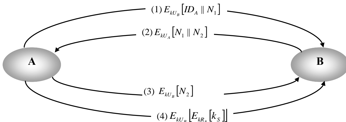
3.6- rasm. Faol va passiv hujumlardan himoyani ta'minlash sxemasi
