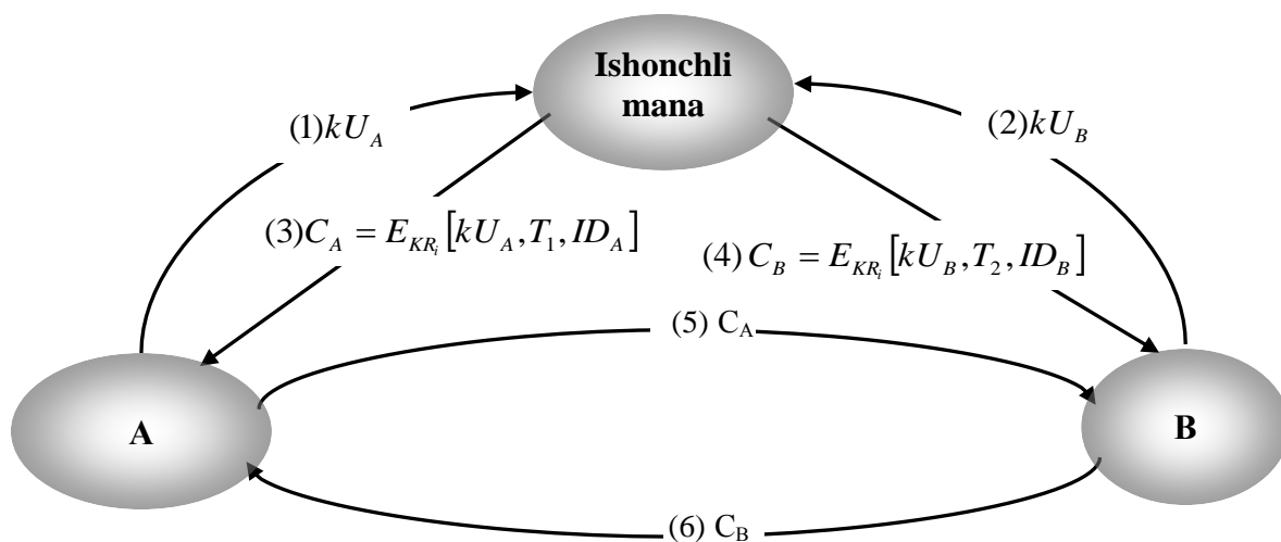
3.4- rasm. Ochiq kalitlar sertifikatlari
