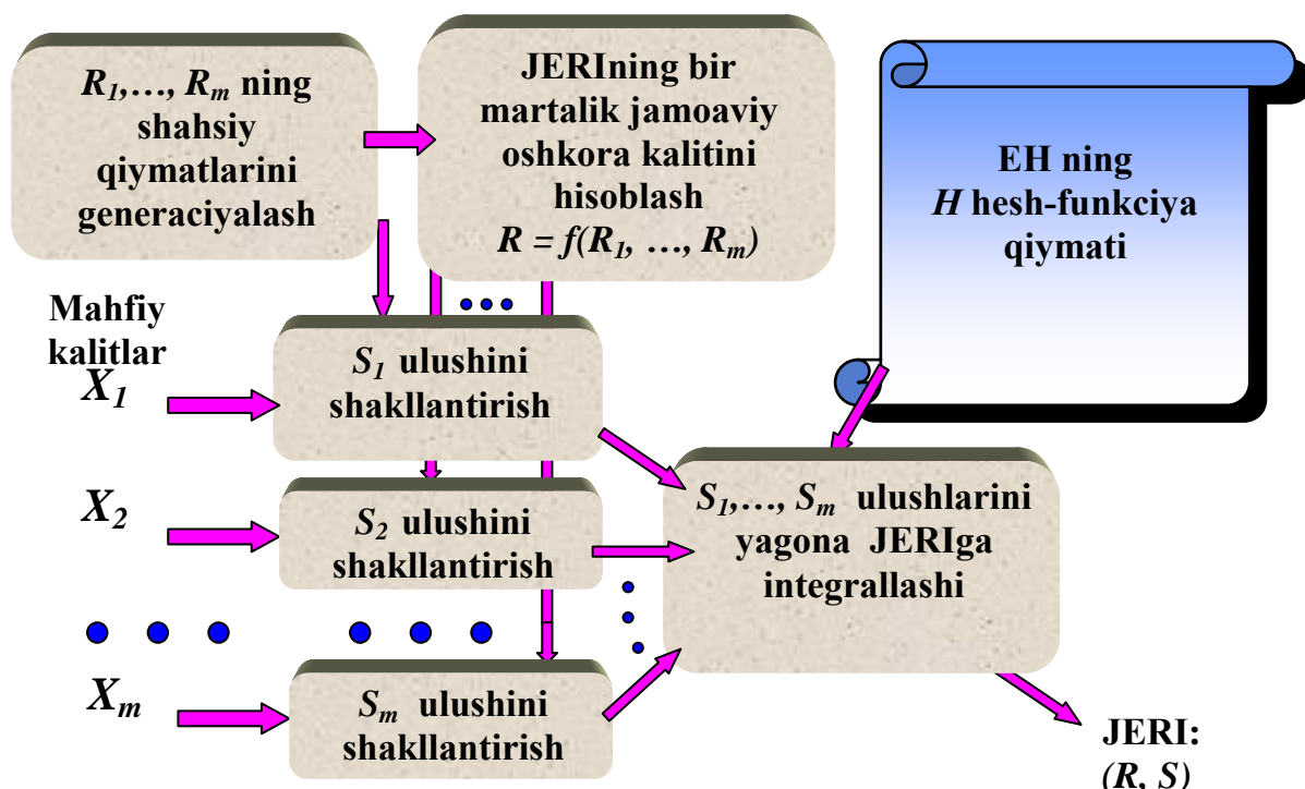
4.3- rasm. JERI shakllantirishning umumiy sxemasi
