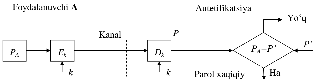
2.1- rasm. Paroldan foydalangan holda oddiy autentifikasiyalash
