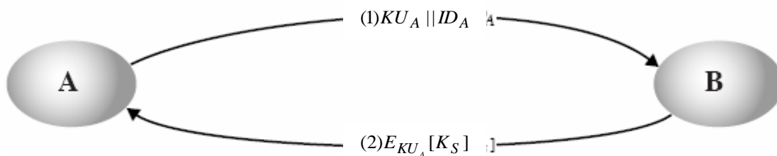
3.5- rasm. Maxfiy kalitlar taqsimlashning Merkel sxemasi
