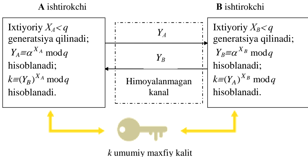
3.15- rasm. Diffi-Xellman sxemasini qoʻllashga doir protokol
