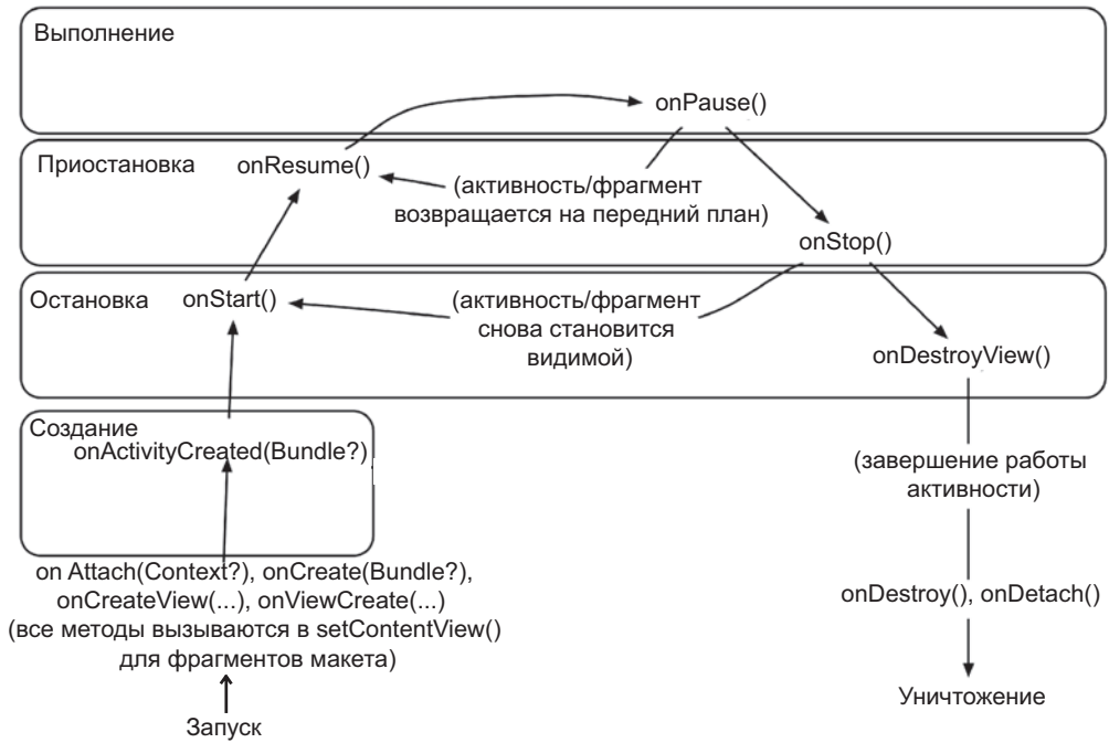
Рис. 8.15. Жизненный цикл фрагмента
