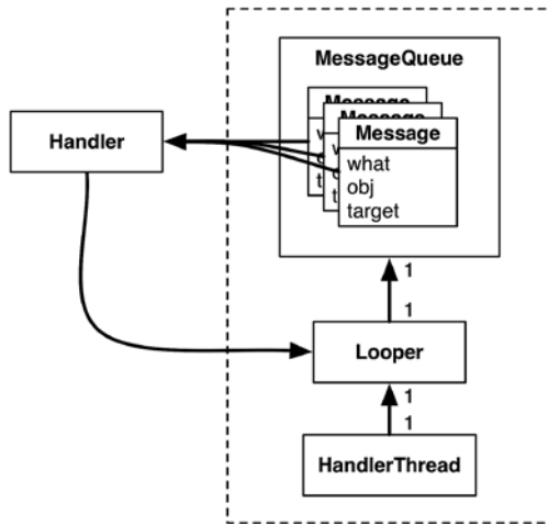
Рис. 25.5. Looper , Handler , HandlerThread и Messages
