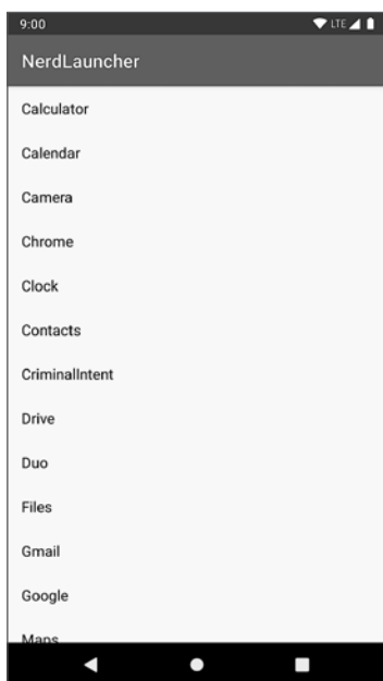
Рис. 23.3. Список activity
