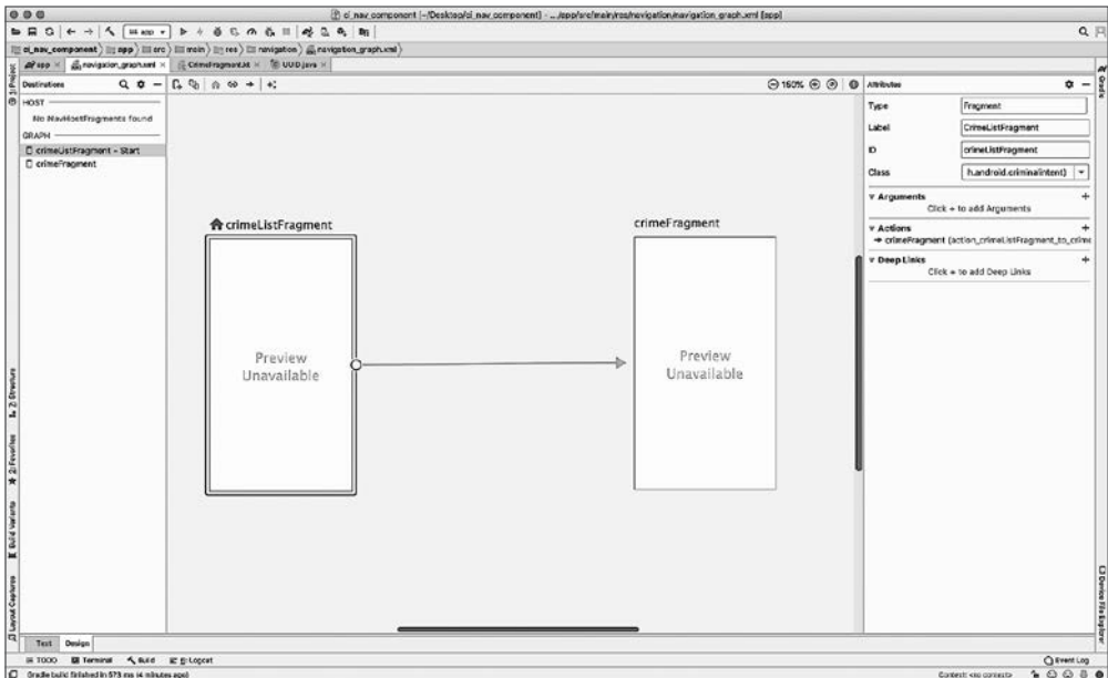
Рис. 12.4. Редактор навигации
