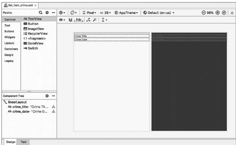
Рис. 10.7. Новый ConstraintLayout
