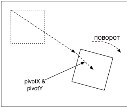
Рис. 31.3. Поворот представления
