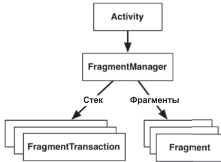
Рис. 8.13. Компонент FragmentManager
