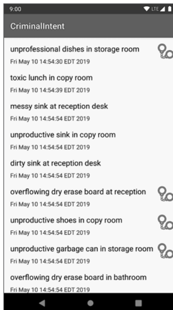
Рис. 14.2. Панель приложения
