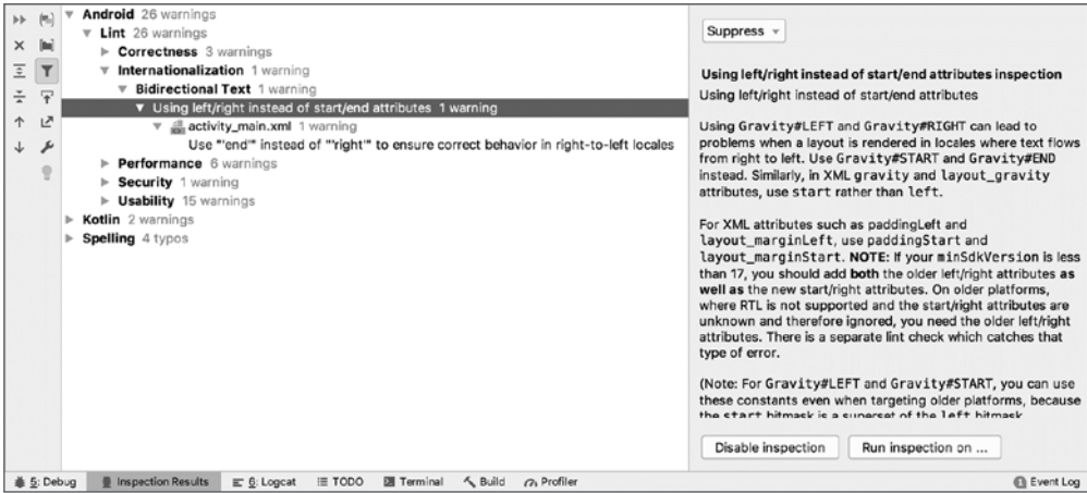
Рис. 5.10. Описание предупреждения
