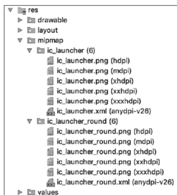
Рис. 22.6. Значки mirmap
