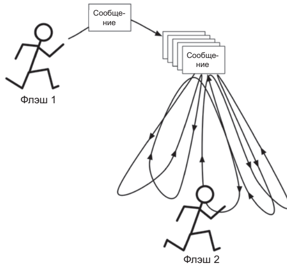
Рис. 25.2. Цикл сообщений
