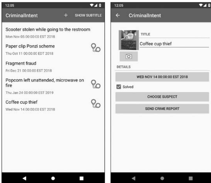
Рис. 8.1. Приложение CriminalIntent
