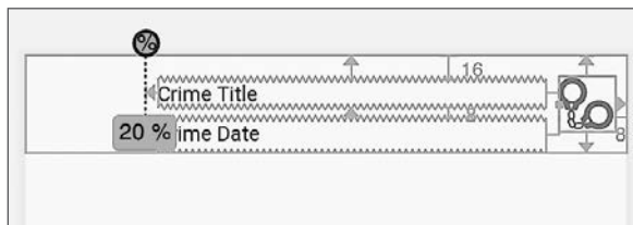
Рис. 10.35. Использование направляющих
