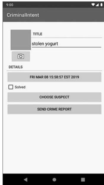
Рис. 16.1. Новый интерфейс
