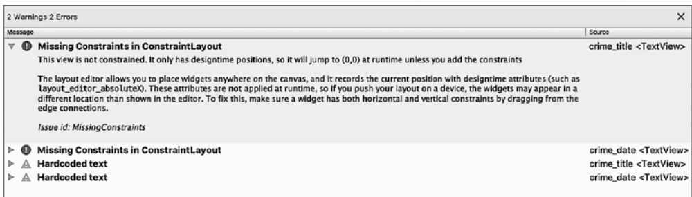
Рис. 10.9. Предупреждения ConstraintLayout
