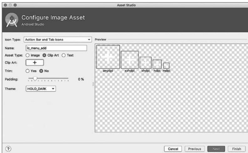
Рис. 14.10. Asset Studio
