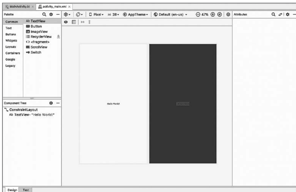
Рис. 1.9. Редактор макета
