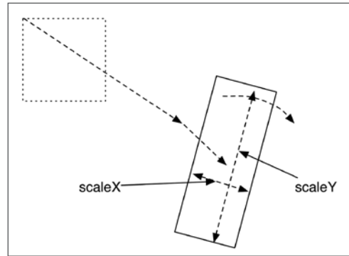
Рис. 31.4. Масштабирование представления
