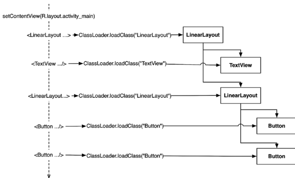
Рис. 1.22. Заполнение activity_main.xml
