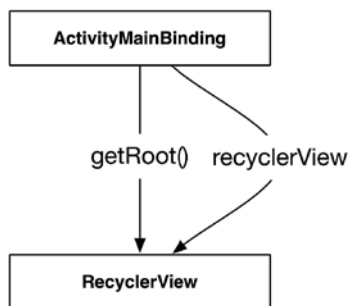
Рис. 19.2. Класс привязки
