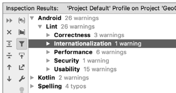
Рис. 5.9. Предупреждения Lint
