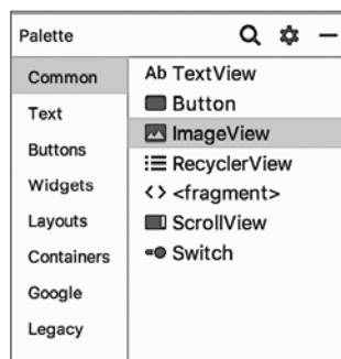
Рис. 10.14. Поиск ImageView
