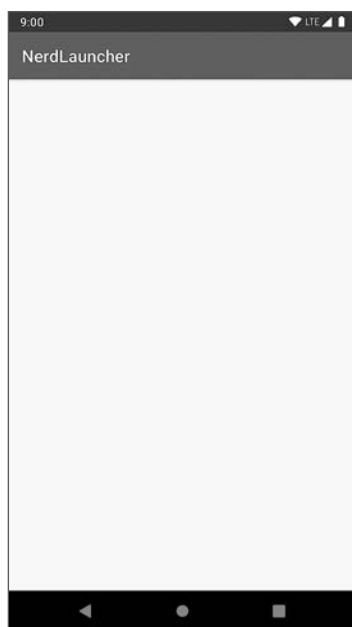
Рис. 23.2. NerdLauncher — начало
