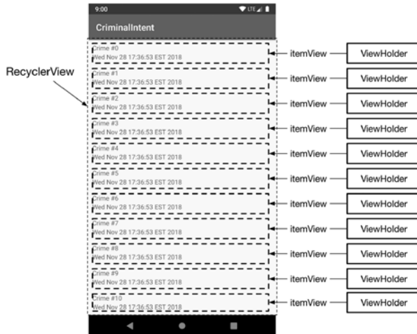
Рис. 9.7. Визуализация ViewHolder
