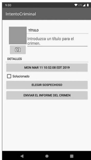
Рис. 17.1. IntentoCriminal
