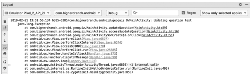
Рис. 5.3. Результаты
