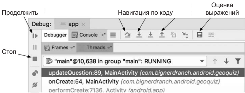
Рис. 5.7. Панель Debug
