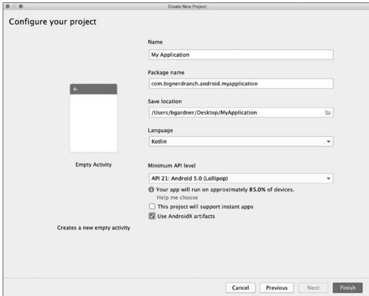
Рис. 4.10. Добавление Jetpack-библиотек
