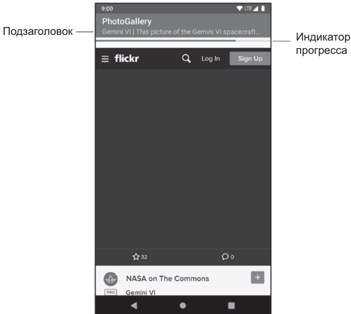
Рис. 29.3. Крутой WebView
