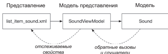
Рис. 19.10. Архитектура MVVM
