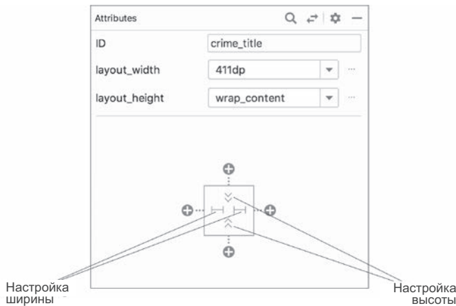
Рис. 10.10. Атрибуты TextView
