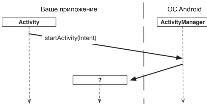
Рис. 6.7. Запуск activity
