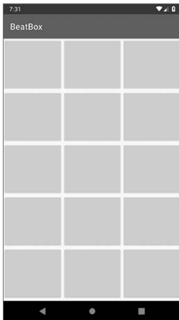
Рис. 19.6. Пустые кнопки
