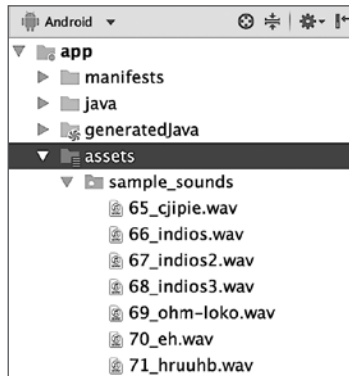
Рис. 19.5. Импортированные активы
