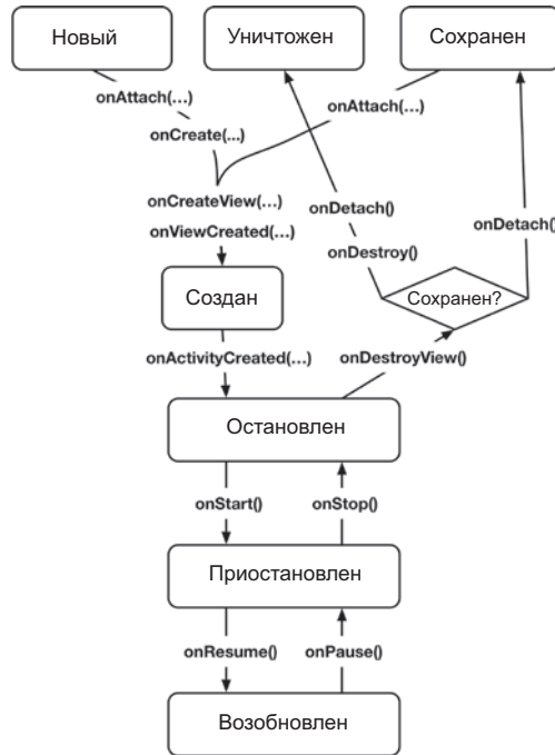
Рис. 25.13. Жизненный цикл фрагмента
