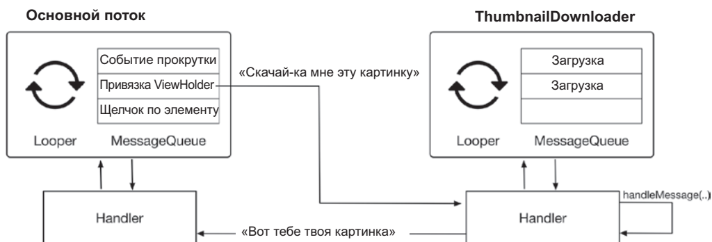
Рис. 25.4. Взаимодействие с обработчиками
