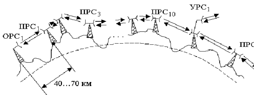
Рис. 4.2. Схематичное представление радиорелейной линии
