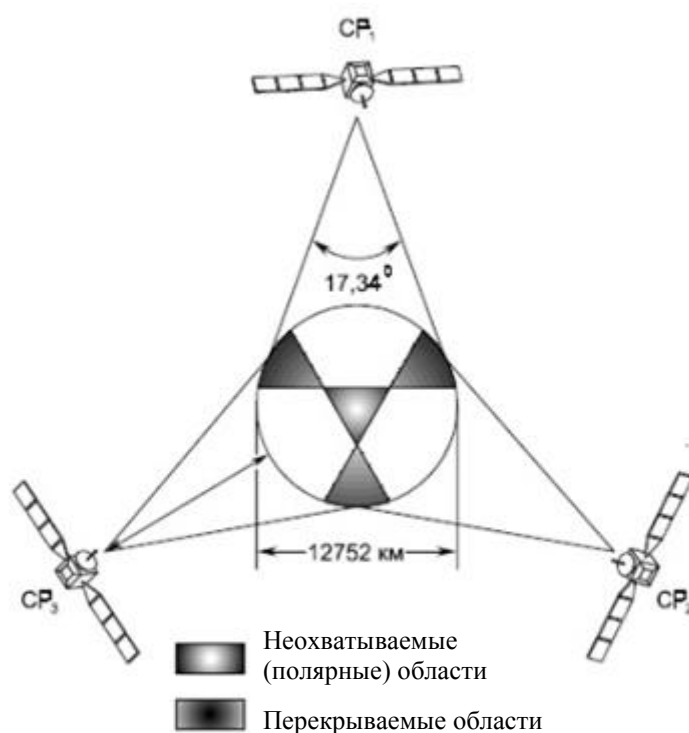
Рис. 4.7. Схема охвата Земли тремя геостационарными спутниками
