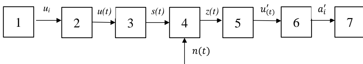
Рис. 1.6. Структурная схема одноканальной системы связи
