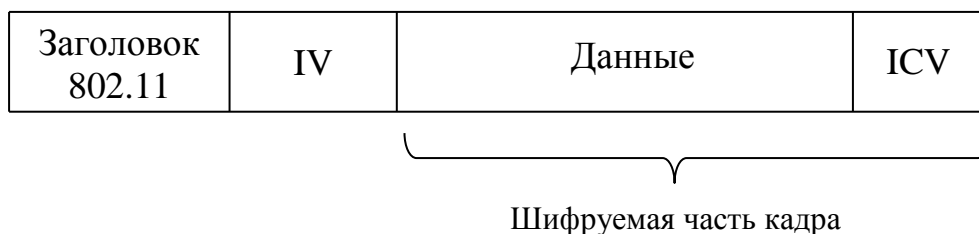
Рис. 8.2. Формат WEP-кадра
