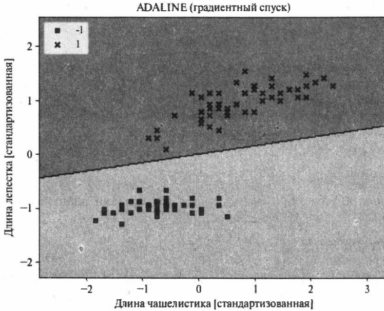
Рис. 4.56. Цветовое выделение областей, разделяющих два вида ирисов на основе стандартизованной обучающей выборки и адаптивного линейного нейрона
