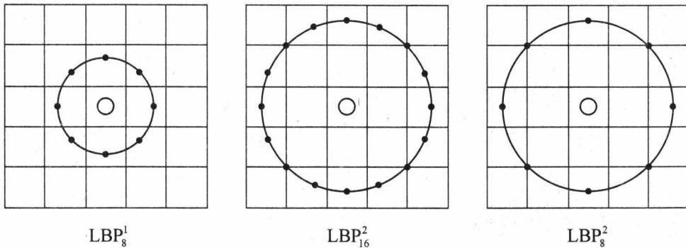
Рис. 8.23. Иллюстрация сущности параметров локальных бинарных шаблонов изображения
