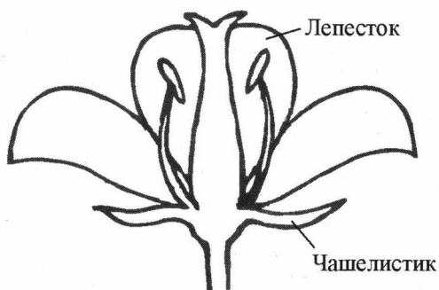
Рис. 4.46. Структура ириса
