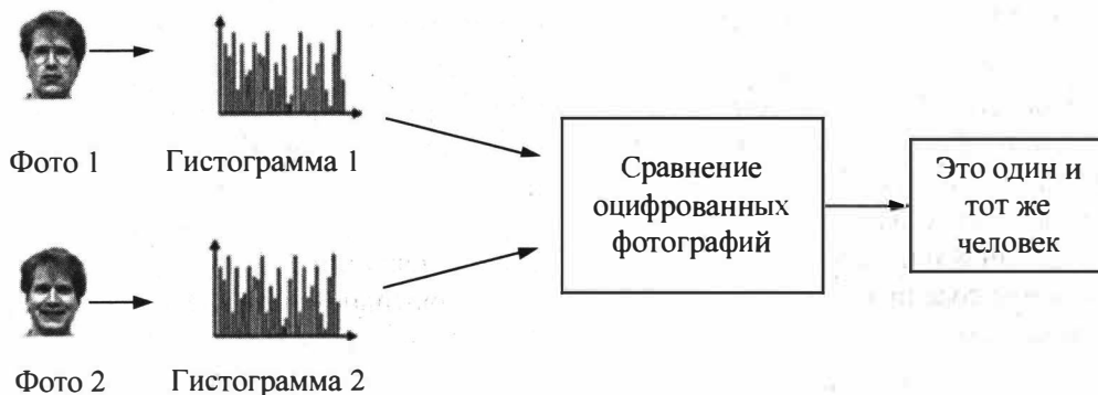
Рис. 8.22. Алгоритм сравнения похожести лиц на основе локальных бинарных шаблонов изображения
