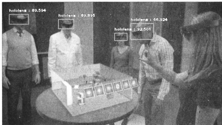
Рис. 7.23. Изображение, полученное на выходе из обученной сети
