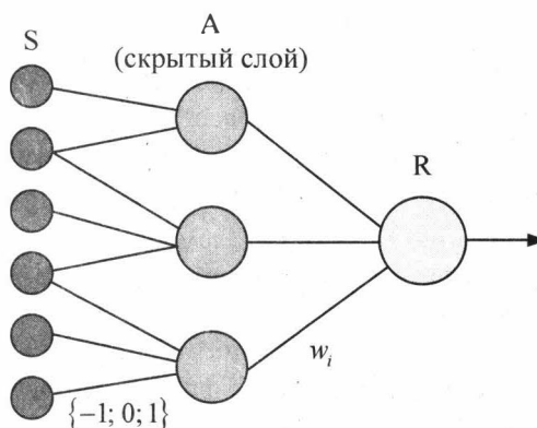
Рис. 4.6. Структура персептрона с одним скрытым слоем
