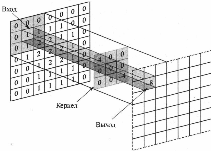
Рис. 6.22. Принцип работы свертки изображения
