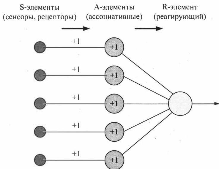
Рис. 4.23. Простейший однослойный перцептрон с одним скрытым слоем
