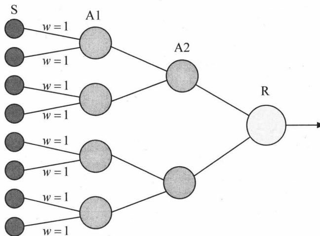
Рис. 4.11. Многослойный перцептрон
