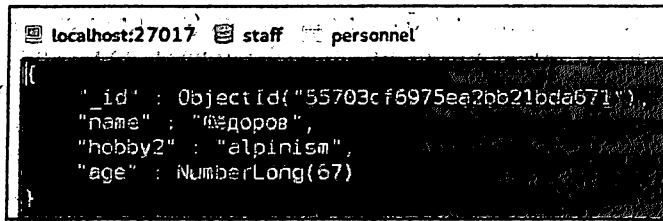
Рис. 8.25. Отображение явно заданного типа данных в документе
