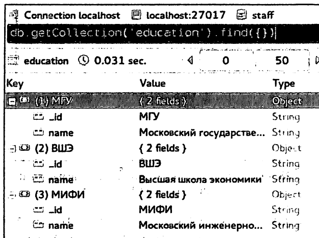
Рис. 8.29. Создание коллекции education
