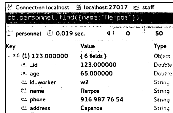
Рис. 8.5. Результат выборки документов с именем «Петров»
