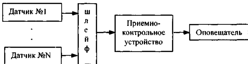
Рис. 4. Структура типовой системы охранной сигнализации
