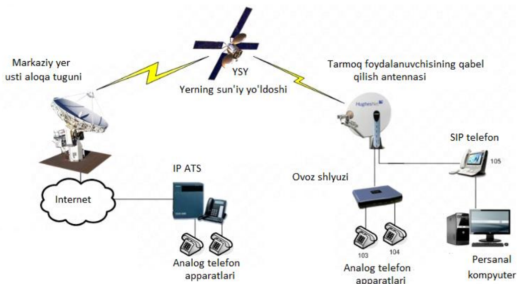
2.3-rasm. Sun'iy yo'ldoshli aloqa tizimining tashkil etilishi
