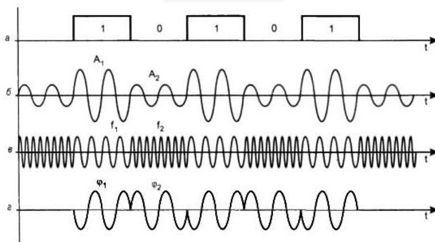
3.8-rasm. Diskret ma'lumotlarni uzatishda qo'llaniluvchi turli hil monipulyatsiya usullari
