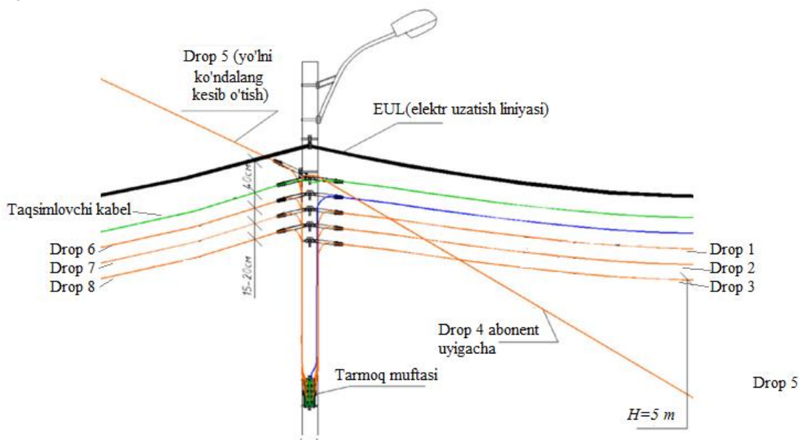
9.10-rasm FTTC havo aloqa liniyasini qurishda optik kabellarni tayanchlarga vertikal usulda osish texnologiyasi qoʻllanilishi
