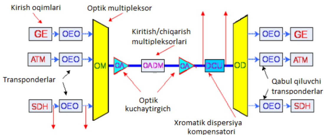
5.7-rasm. DWDM texnologiyasining ishlash tamoyilini tushuntiruvchi sxemasi
