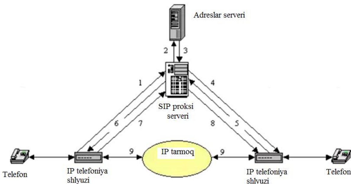
8.3-rasm. SIP protokolining IP tarmoq orqali telefaniya’ni ta‘minlashda qo‘llanilishi
