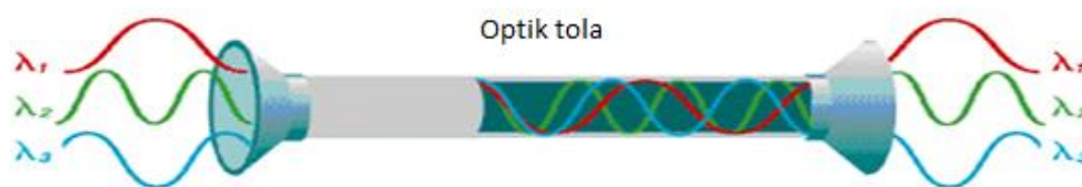
5.2-rasm. Bir optik tola orqali bir necha alohida to'lqin uzunliklaridagi aloqa kanallari tashkil qilinishi
