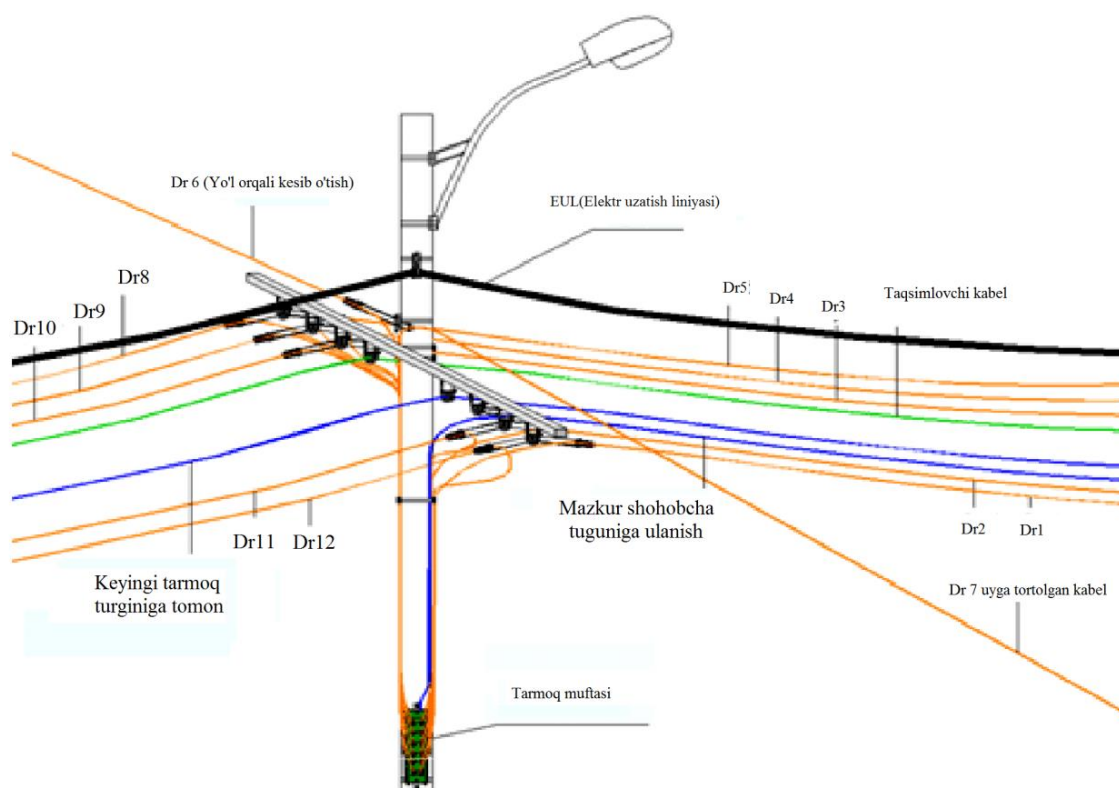
9.11-rasm Osiluvchi trosdarga birlashtirish usulida optik kabelli havo aloqa liniyasini qurish
