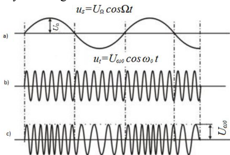
3.4-rasm. Chastota boʻyicha modulyatsiya jarayoni
