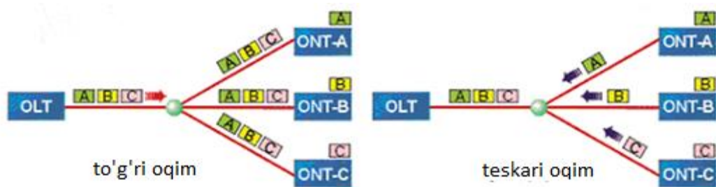
4.20-rasm. PON tarmog'ida to'g'ri va teskari oqimning yuzaga kelishi.
