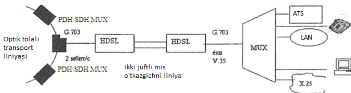
4.7-rasm. HDSL texnologiyasi asosidagi abonent ulanish liniyasi
