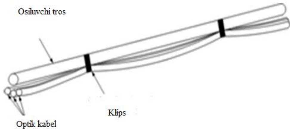
9.12-rasm. Aloqa kabellarini trosga birlashtirishda klips yoki tortma usuli
