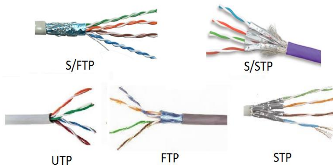
2.4-rasm. Simmetrik o`rama juftli kabellarning turlari
