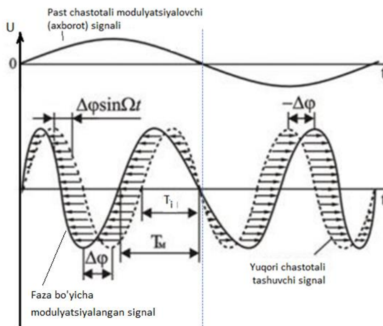
3.6 – rasm. Tashuvchini faza bo'yicha modulyatsiyalash jarayoni
