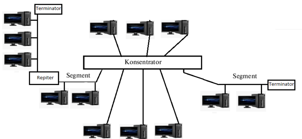
6.1 – rasm. Ethernet tarmogʻi va unda tarmoq elementlarining ulanish topologiyasi
