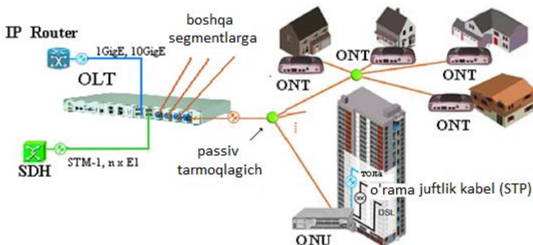
4.15-rasm. PON texnologiyasi asosida qurilgan passiv optik tarmoqning prinsipial sxemasi
