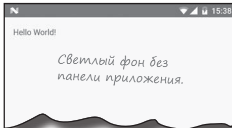
Theme.AppCompat.Light.NoActionBar
