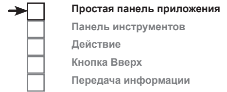
Theme.AppCompat
