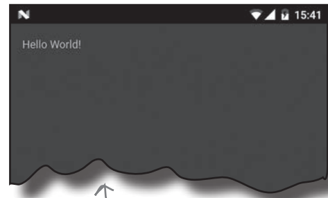
Theme.AppCompat.NoActionBar
