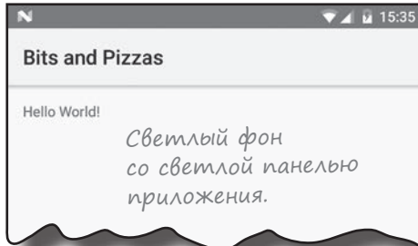
Theme.AppCompat.Light
