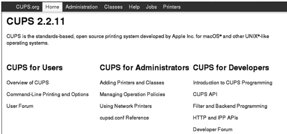
Рис. 16.1. Веб-администрирование CUPS
