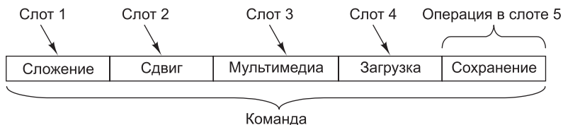
Рис. 8.3. Стандартная TriMedia-команда с пятью операциями
