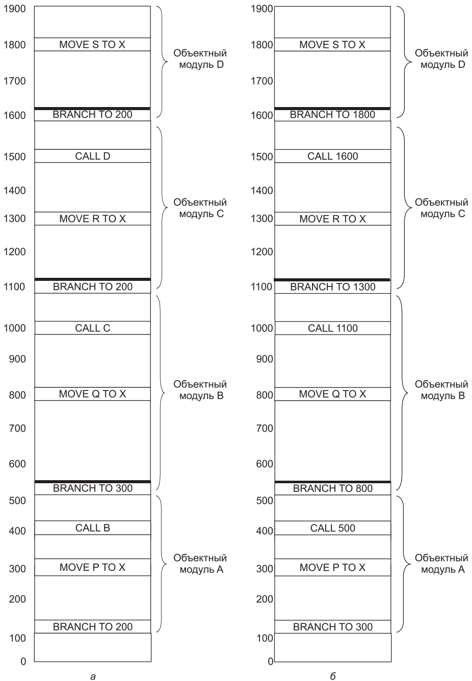
Рис. 7.4. Объектные модули после размещения в двоичном образе, но до перераспределения памяти и компоновки ( а ); те же объектные модули после компоновки и перераспределения памяти ( б ). В результате получается исполняемый двоичный код, который можно запускать
