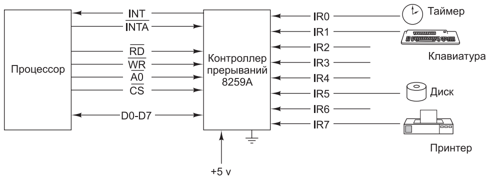
Рис. 3.40. Контроллер прерываний 8259А
