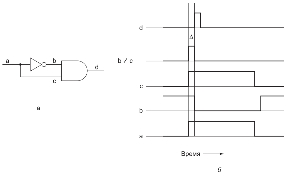
Рис. 3.23. Генератор импульса ( a ); временная диаграмма для четырех точек на схеме ( b )
