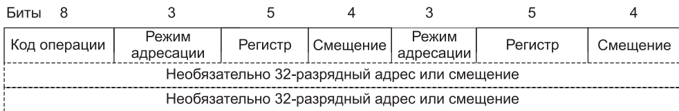
Рис. 5.17. Простые форматы команд для двухадресной машины
