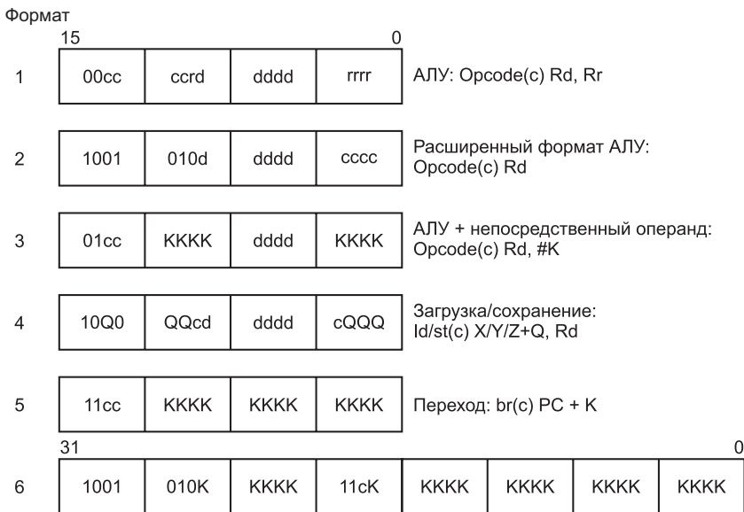
Рис. 5.11. Форматы команд ATmega168 AVR
