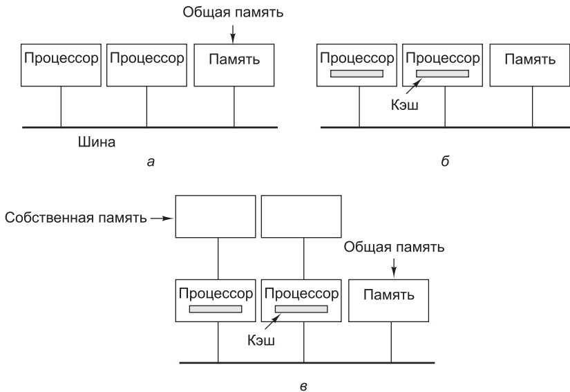
Рис. 8.23. Три варианта мультипроцессора на одной шине: без кэш-памяти ( а ); с кэш-памятью ( б ); с кэш-памятью и отдельными модулями локальной памяти ( в )
