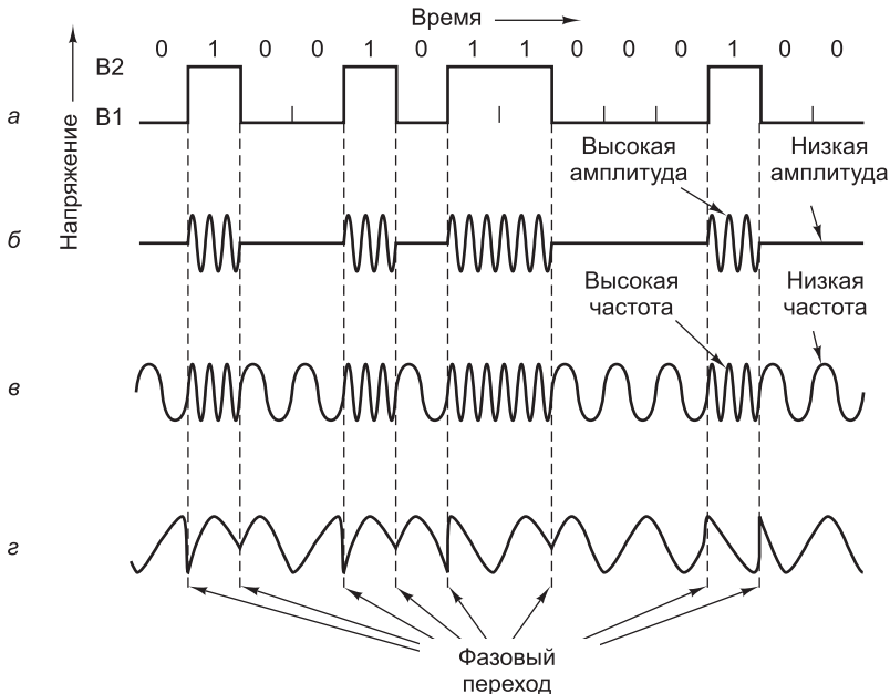
Рис. 2.34. Последовательная передача двоичного числа 01001011000100 по телефонной линии: двухуровневый сигнал ( a ); амплитудная модуляция ( b ); частотная модуляция ( в ); фазовая модуляция ( г )
