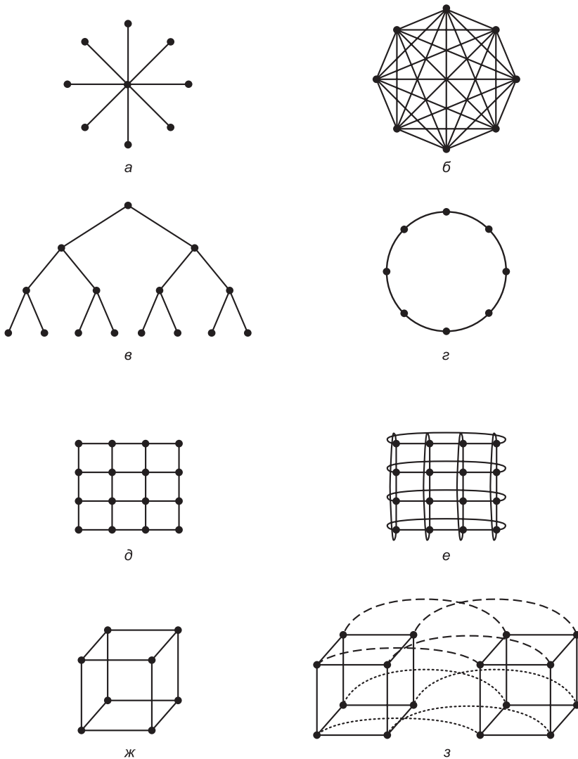
Рис. 8.33. Различные топологии. Жирные точки соответствуют коммутаторам. Процессоры и модули памяти не показаны: звезда (а); полная взаимосвязь (б); дерево (в); кольцо (г); решетка (д); двойной тор (е); куб (ж); четырехмерный гиперкуб (з)
