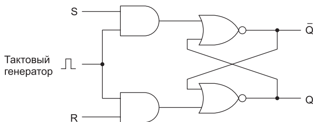
Рис. 3.21. Синхронная SR-защелка
