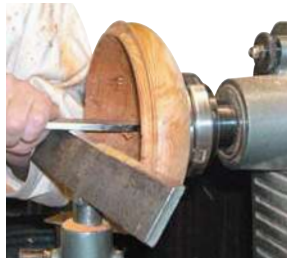
车削 chēxiāo | turn (v)
