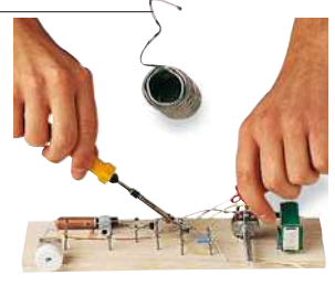
焊接 hànjiē | solder (v)
