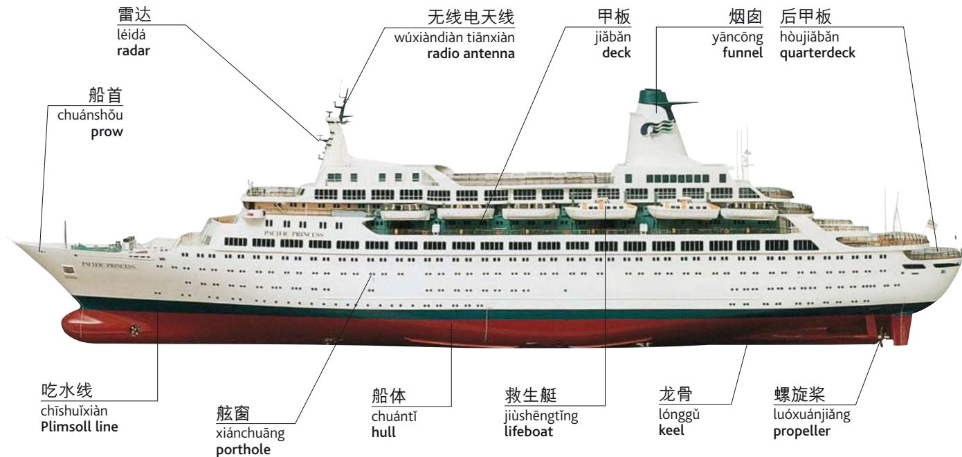
远洋客轮 yuǎnyángkèlún | ocean liner
