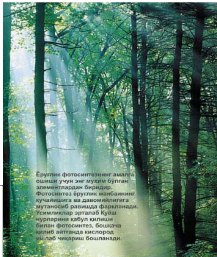
Ёруғлик эгри чизигига фотосинтезнинг реакцияси
