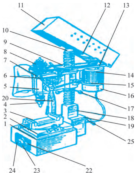
47-rasm. Parmash dastgohi.
