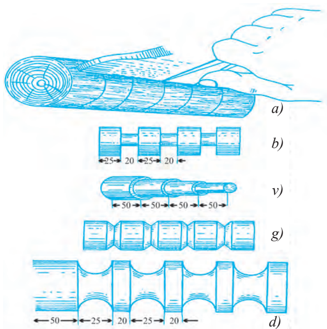
17-rasm. Turli xil sirtlarni rejalash va yo'nish: a – sirkul yordamida rejalash; b – tik bo'yinlar hosil qilish; v – pog'onali sirtlar; g – o'yiqlar; d – botiq sirtlar.
