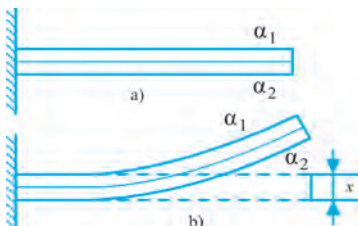
54-rasm. Bimetall yaproqni haroratga bog‘liqlik holati
