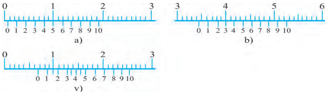
33-rasm. Shtangensirkul shkalalarining o'lchashdagi holatlari: a) 0,5 mm; b) 6,9 mm; v) 34,3 mm
