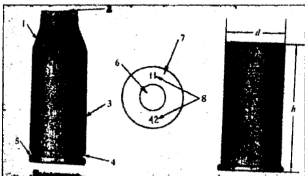
15-расм, Гилза турлари, (Бутилка ва цилиндр шаклида) рақамлар билан отишдан қоладиган белгилар кўрсатилган
