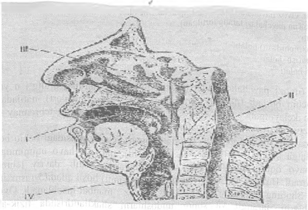
5-rasm. Boshning bo'ylama kesmasi. Yumshoq tanglay pastga tomon siljigan. I. Og'iz bo'shlig'i. II. Halqum. III. Burun bo'shlig'i. IV. Bo'g'iz 29 .
