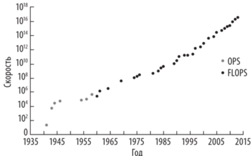
Рис. 3. Производительность сверхмощных компьютеров. В прямом смысле то, что называют «закон Мура», – это наблюдение, согласно которому количество транзисторов, размещаемых на кристалле интегральной схемы, удваивается примерно каждые два года. Однако часто закон обобщают, считая, что так же по экспоненте растут и другие показатели производительности компьютеров. На нашем графике показано изменение во времени пиковой скорости наиболее сверхмощных компьютеров в мире (по логарифмической вертикальной шкале). В последние годы скорость последовательных вычислений расти перестала, но за счет распространения параллельных вычислений общее количество операций продолжает увеличиваться с прежним темпом 16 .
